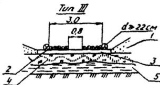
Графическая схема 2. Усиление ледовых переправ деревянным настилом: 1 - снеговой покров; 2 - колесопроеды; 3 - поперечины; 4 - естественный ледяной покров; 5 - вода
